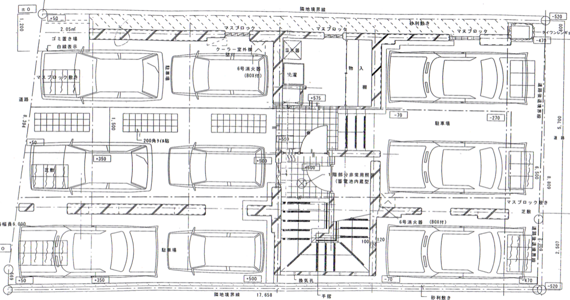
1階平面図
