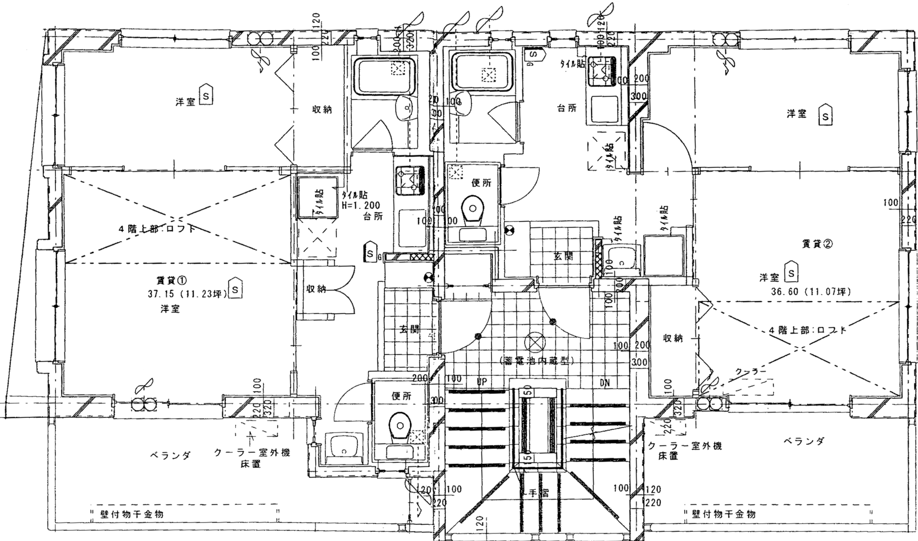
3・4階平面図
