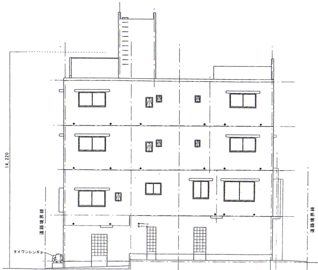
西立面図
